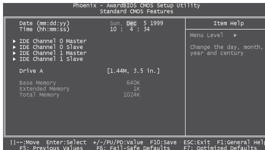
基本 CMOS 参数设置
