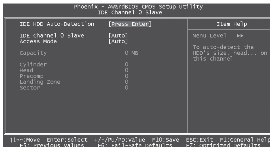
第一主硬盘设置菜单
