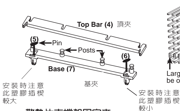
散熱片支撐架固定夾
