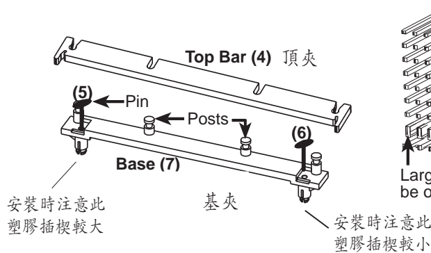
散熱片支撐架固定夾
