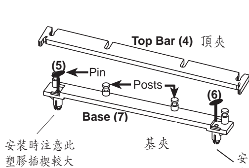
散熱片支撐架固定夾
