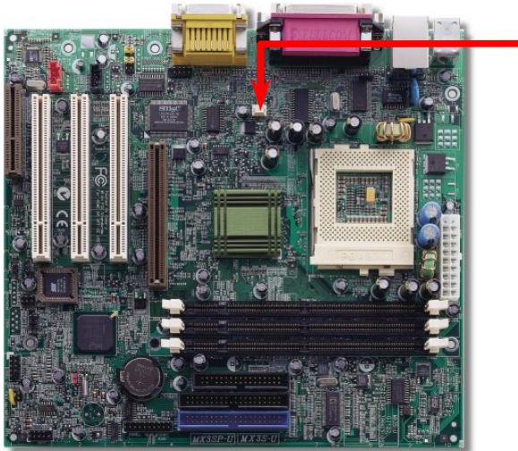
CPU Fan Connector
