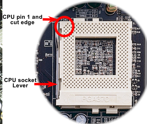
CPU cut edge
