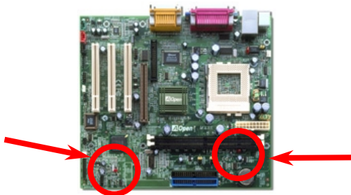
LED Alimentazione RAM
