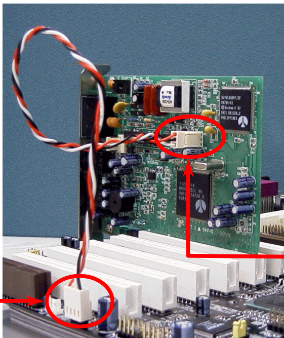
WOM接頭(主機板端)
