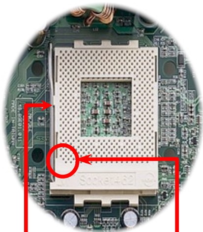
CPU 插座固定桿
