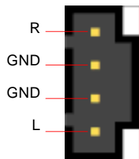
CD 音源接頭
