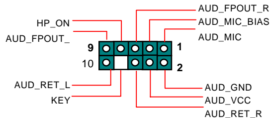
主機板前方面板音效擴接接頭
