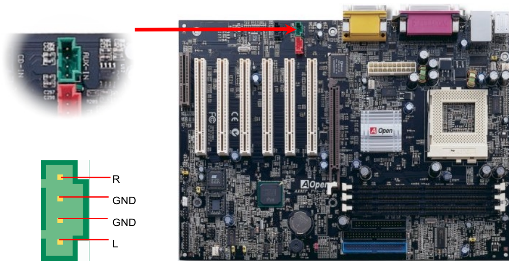
AUX 入力
