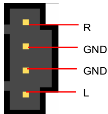
CD 入力
