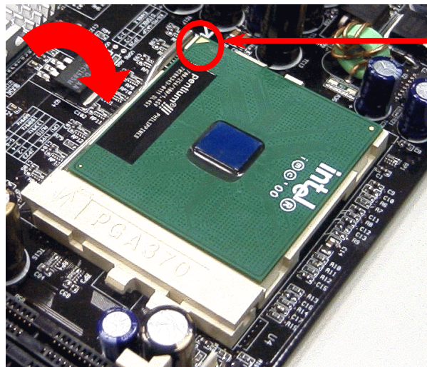
Encoche CPU
