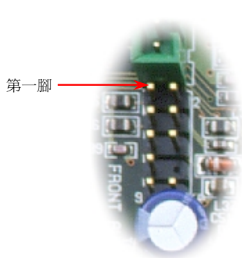
主機前方面板音效擴接接腳
