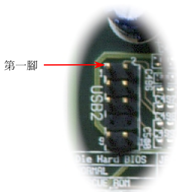
第二組 USB 連接埠接腳
