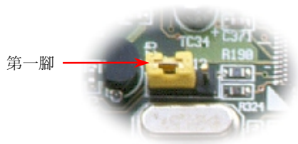
JP12 開啓/關閉主機板內建音效跳線
