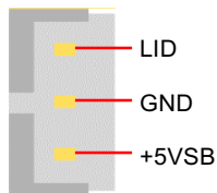
WOL コネクタ
