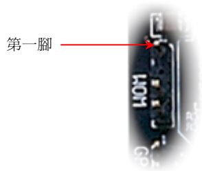
WOM 接腳
