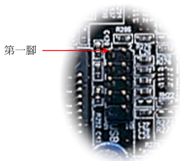
USB2 接頭
