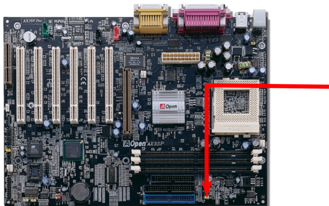
JP23 FSB 選擇跳線
